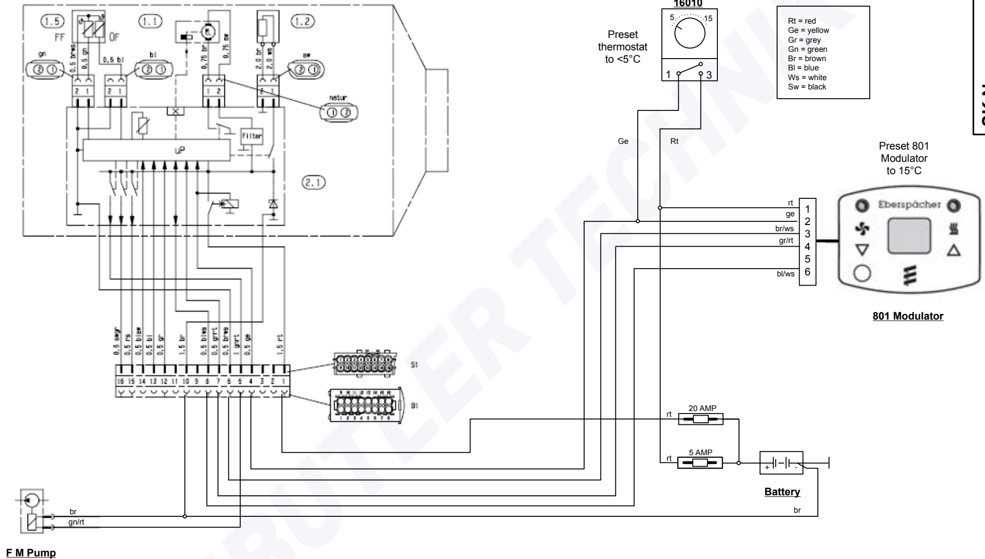
Circuit diagram – AIRTRONIC D2 / AIRTRONIC D4
