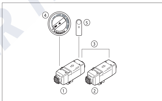
Fig. 01: Systemaufbau
